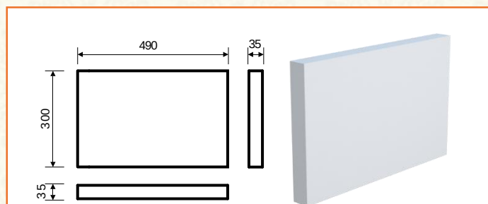
Р-5/4 (300x35x490) Прямой / Угловой
