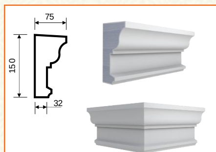
T-3 (150x75x2000)
