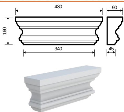
Кпл-4 (160х90х430) прямая/угловая
