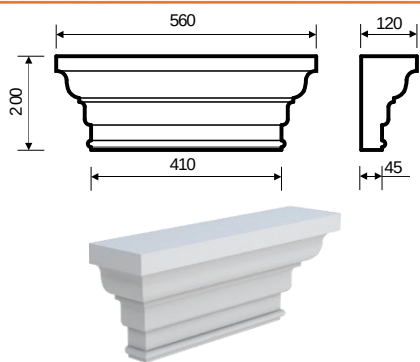
Кпл-3 (200х120х560) прямая/угловая
