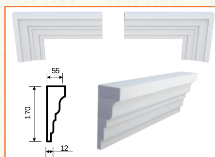
M-42 (170x55x2000)
