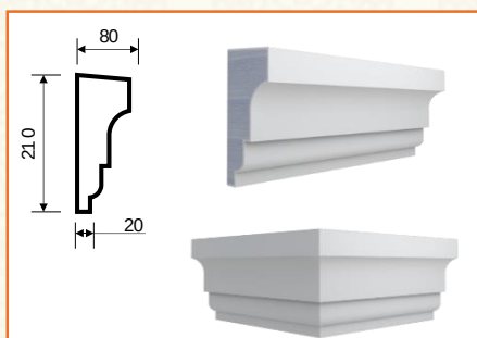
T-23 (210x80x2000)
