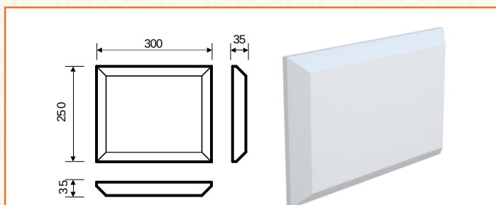
Р-1/1 (250x35x300) Прямой / Угловой
