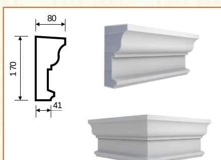
T-17 (170x80x2000)
