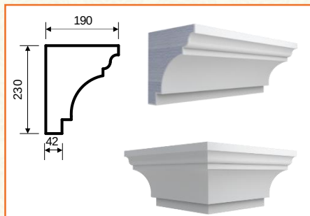
K-16 (230x190x2000)
