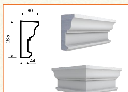
T-21 (185x90x2000)
