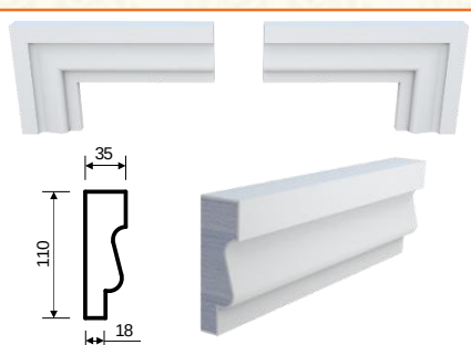
M-10 (110x35x2000)
