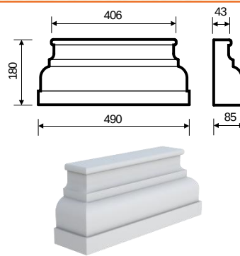
Бпл-3 (180х85х490) прямая/угловая
