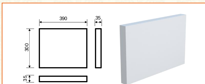
Р-5/3 (300x35x390) Прямой / Угловой
