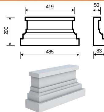
Бпл-2 (200х83х485) прямая/угловая
