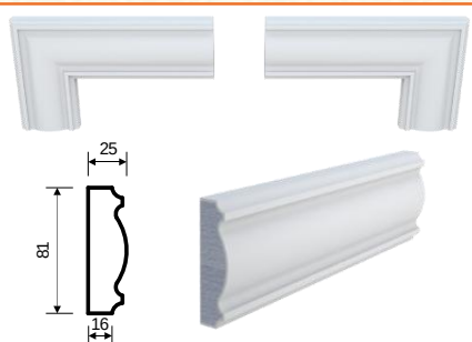
M-4 (81x25x2000)
