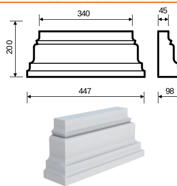
Бпл-4 (200х98х447) прямая/угловая
