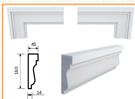
M-41 (160x45x2000)
