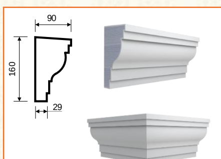
T-16 (160x90x2000)
