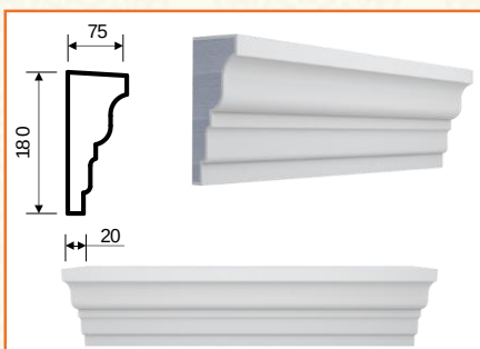
П-11 (180x75x2000)
