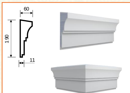
T-10 (190x60x2000)
