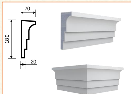
T-7 (180x70x2000)
