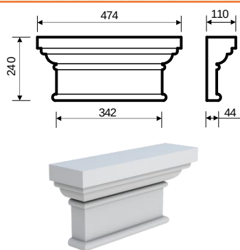
Кпл-2 (240х110х474) прямая/угловая
