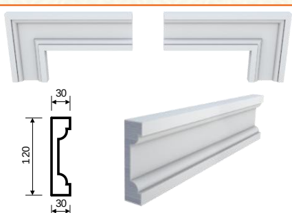
M-13 (120x30x2000)
