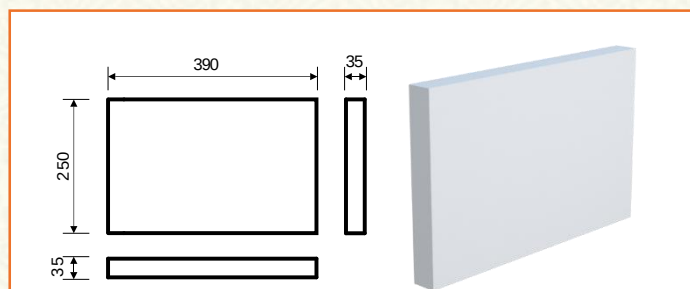
Р-5/2 (250x35x390) Прямой / Угловой
