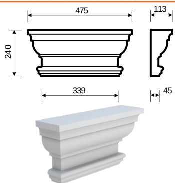
Кпл-1 (240х113х475) прямая/угловая
