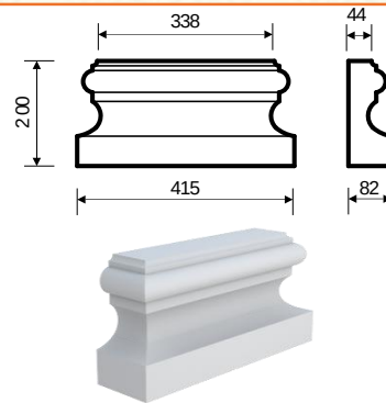
Бпл-1 (200х82х415) прямая/угловая
