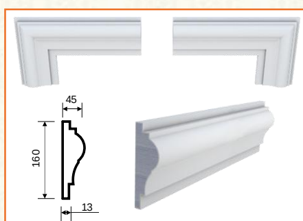
M-40 (160x45x2000)
