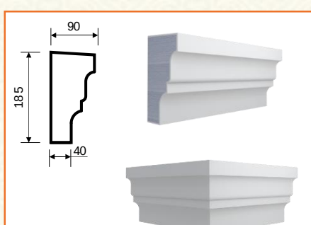
T-20 (185x90x2000)
