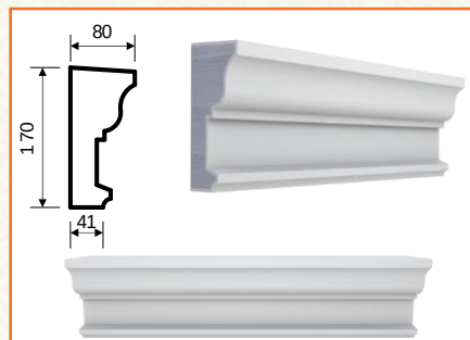
П-15 (170x80x2000)
