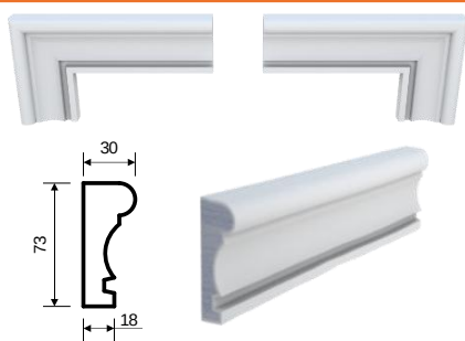
M-2 (73x30x2000)
