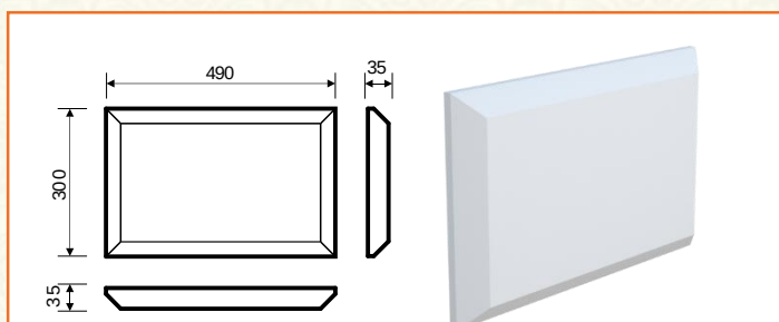
Р-1/3 (300x35x490) Прямой / Угловой
