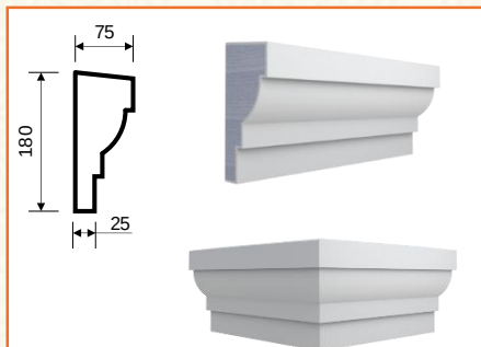
T-8 (180x75x2000)
