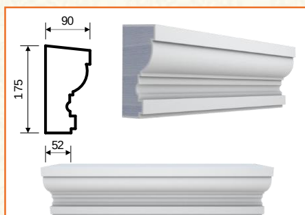
П-16 (175x90x2000)
