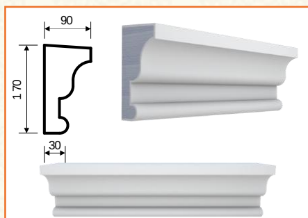
П-10 (170x90x2000)
