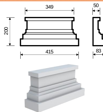
Бпл-2 (200х83х415) прямая/угловая
