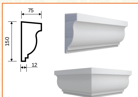
T-4 (150x75x2000)
