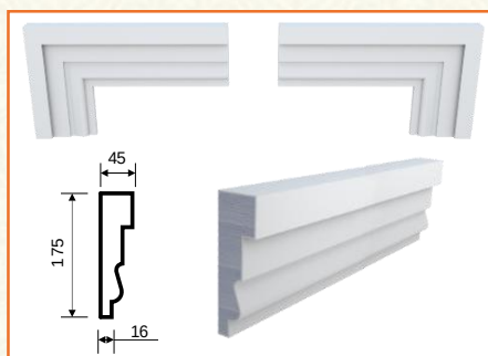
M-43 (175x45x2000)
