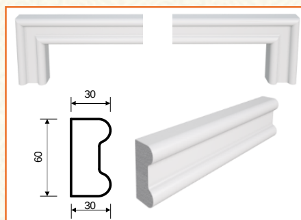
M-44 (60x30x2000)
