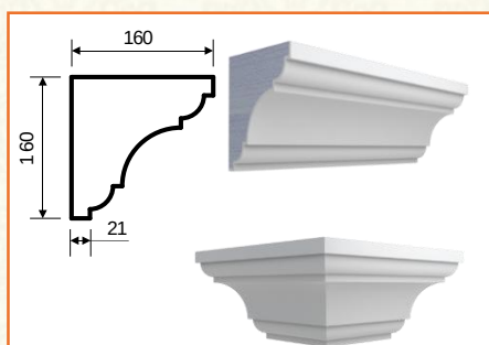
К-4 (160x160x2000)
