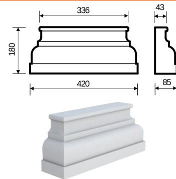
Бпл-3 (180х85х420) прямая/угловая
