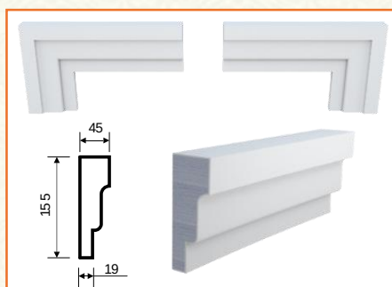
M-37 (155x45x2000)
