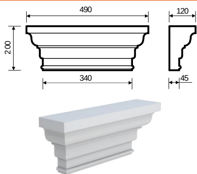
Кпл-3 (200х120х490) прямая/угловая
