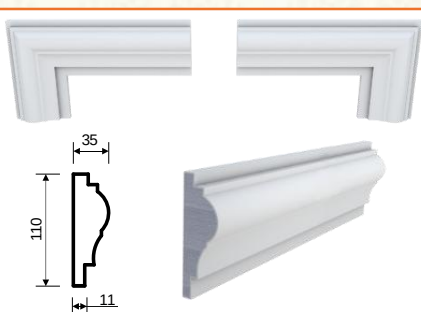
M-11 (110x35x2000)
