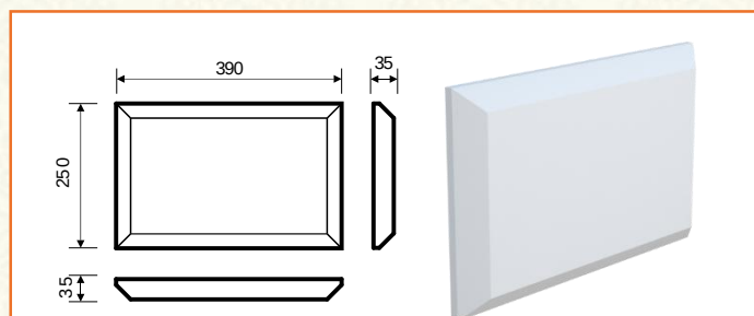
Р-1/2 (250x35x390) Прямой / Угловой
