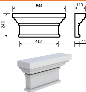
Кпл-2 (240х110х544) прямая/угловая
