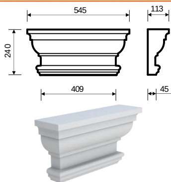
Кпл-1 (240х113х545) прямая/угловая
