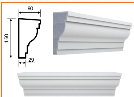
П-14 (160x90x2000)
