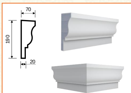
T-22 (190x70x2000)
