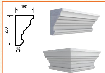
K-19 (250x150x2000)
