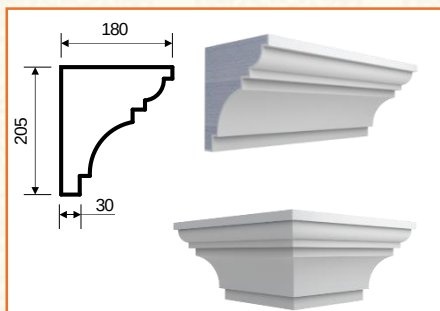
K-14 (205x180x2000)
