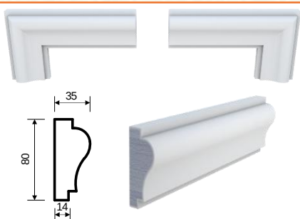
M-5 (80x35x2000)
