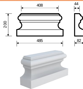
Бпл-1 (200х82х485) прямая/угловая
