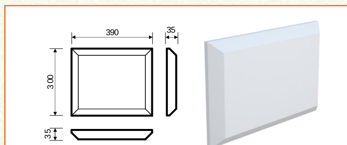
Р-1/4 (300x35x390) Прямой / Угловой
