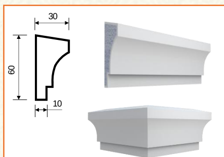
T-1 (60x30x2000)
