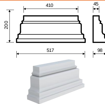
Бпл-4 (200х98х517) прямая/угловая
