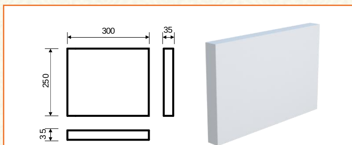
Р-5/1 (250x35x300) Прямой / Угловой
