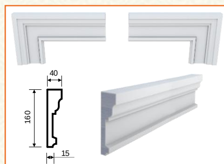
M-39 (160x40x2000)
