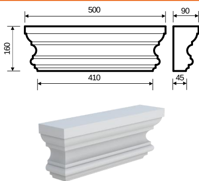
Кпл-4 (160х90х500) прямая/угловая
